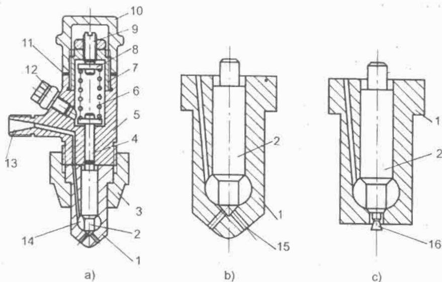
Hình 5-24. Vòi phun
