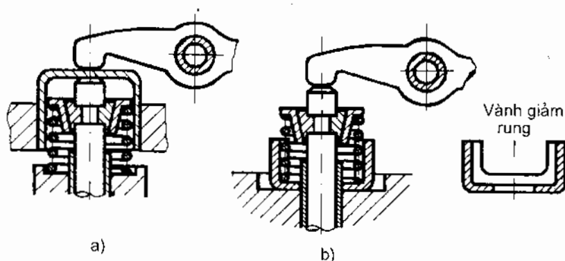
Hình 4-16. Các biện pháp tránh cộng hưởng lò xo xupap bằng giảm chấn
