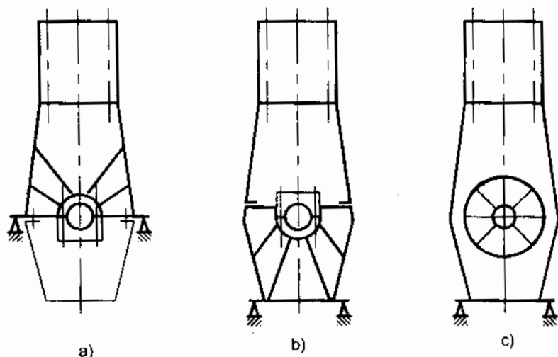
Hình 3-5. Các kiểu lắp đặt trực khuỷu a) trực khuỷu treo, b) trực khuỷu đặt, c) trực khuỷu luồn
