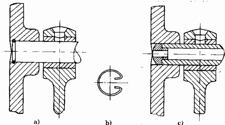
Hình 2-12. Lắp tự do chốt piston
