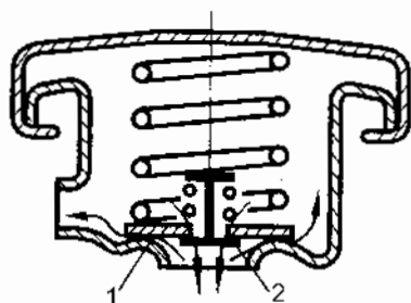
Hình 7-5. Nắp kết nước 1. van xả, 2. van hút
