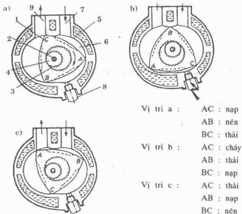
Hình 1.13. Nguyên lý làm việc của động cơ piston quay
