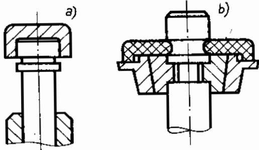
Hình 4-13. Kết cấu ngăn dầu ở đuôi xupap
