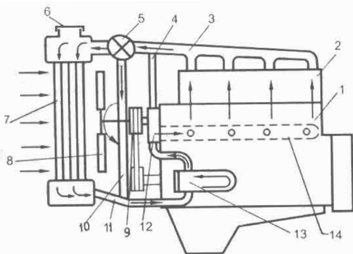
Hình 7-3. Hệ thống làm mát cưỡng bức tuần hoàn kín một vòng
