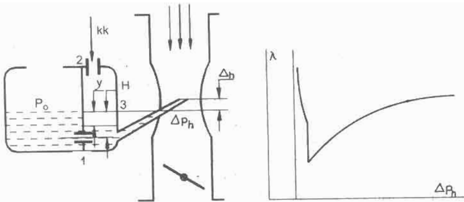
Hình 5-4. Hệ thống chỉnh giảm độ chân không sau giclô chính
