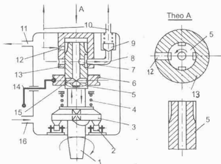
Hình 5-23. Bơm phân phối
