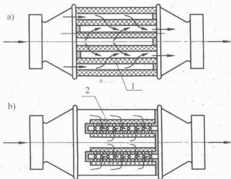
Hình 10-7. Lọc muội than trong khí thải động cơ diesel.
