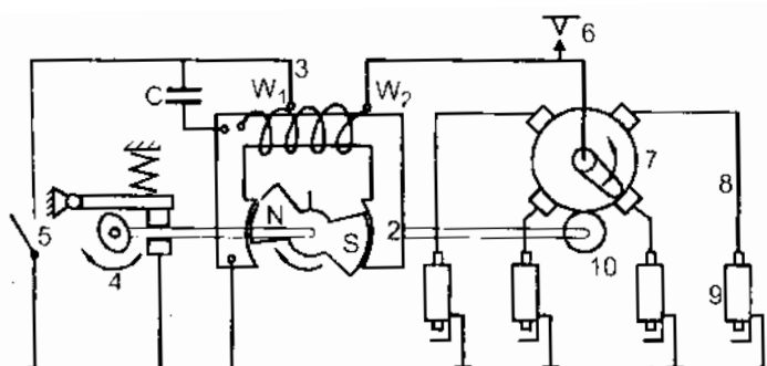
Hình 8-2. Hệ thống đánh lửa bằng nam châm
