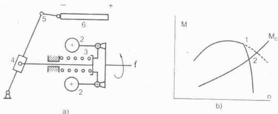
Hình 5-37. Cơ cấu điều tốc kiểu Watt 1. trục điều tốc, 2. quả nặng, 3. lò xo, 4. khớp trượt, 5. thanh nối, 6. thanh răng bơm cao áp
