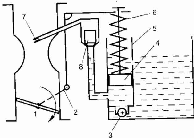
Hình 5-13. Hệ thống tăng tốc 1. bướm ga, 2. đòn dẫn động, 3. van bi, 4. piston, 5. xylanh, 6. lò xo, 7. vòi phun, 8. van rai
