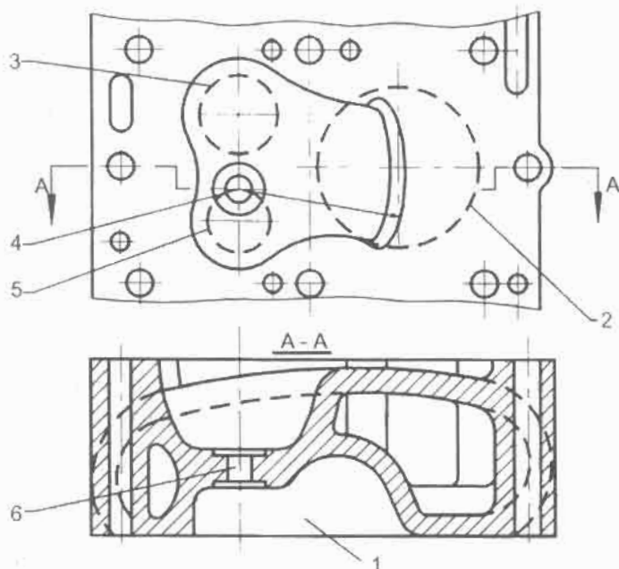
Hình 3-8. Nắp xylanh với buồng cháy Ricardô
