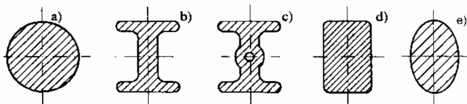
Hình 2-19. Các loại tiết diện thân thanh truyền
