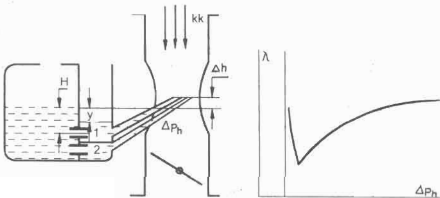
Hình 5-5. Hệ thống chỉnh là giclô bổ sung
