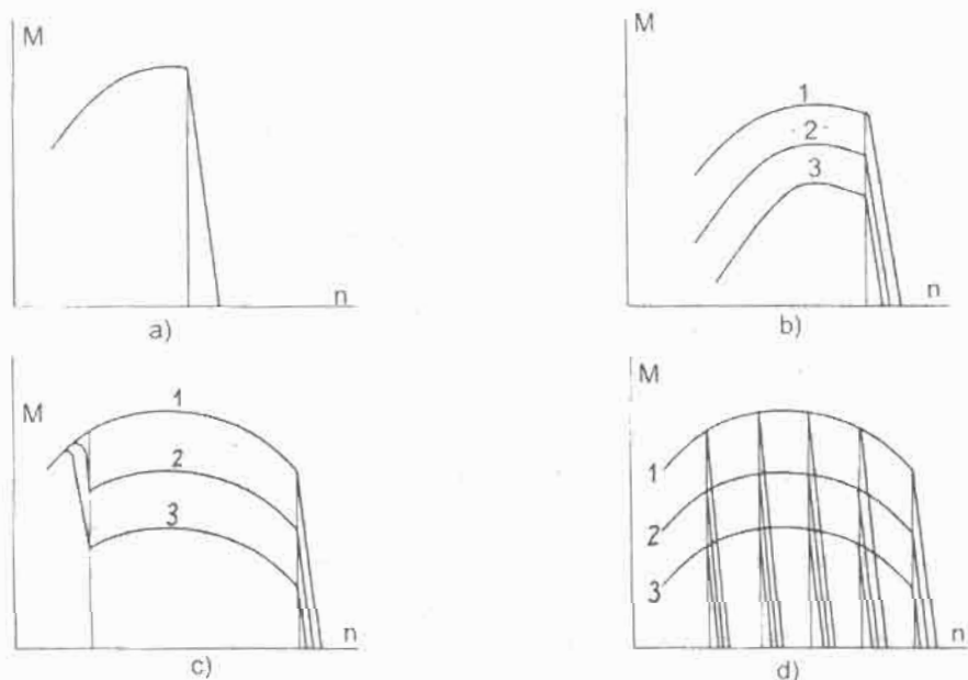
Hình 5-38. Đặc tính động cơ với các loại điều tốc a) điều tốc một chế độ, b) điều tốc giới hạn, c) điều tốc hai chế độ, d) điều tốc đa chế độ
