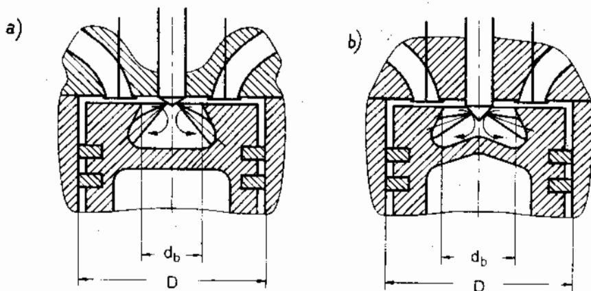
Hình 5-32. Buồng cháy với hỗn hợp thể tích-màng
