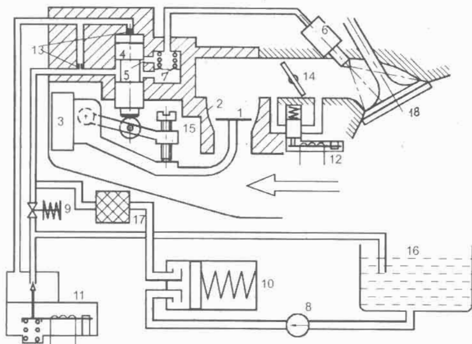
Hình 5-18. Hệ thống phun xăng K - Jetronic
