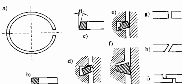
Hình 2-14. Kết cấu xecmăng khí
