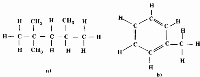
Hình 1-3. Sơ đồ cấu tạo phân tử : a) isooctan \text{C}_8\text{H}_{18} và b) metylbenzen \text{C}_6\text{H}_5\text{CH}_3
