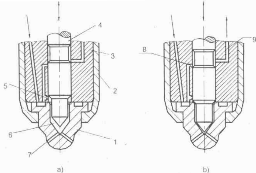
Hình 5-25. Bơm cao áp - vòi phun
