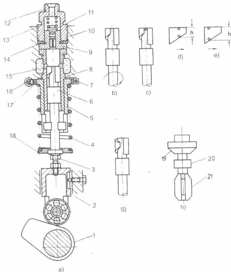
Hình 5-22. Bơm cao áp đơn kiểu Bosh
