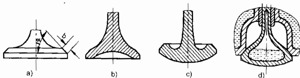
Hình 4-6. Kết cấu nấp xupap
