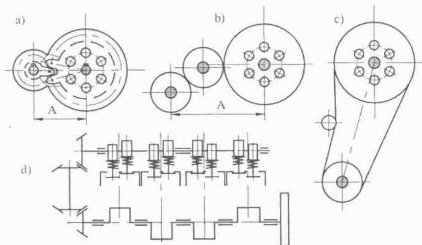
Hình 4-4. Dẫn động trực cam
