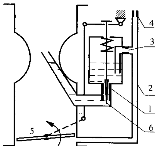
Hình 5-7. Hệ thống chính thay đổi tiết diện gicơ kết hợp với hệ thống không tải. 1. gicơ chính, 2. ống hỗn hợp của hệ thống không tải, 3. gicơ không tải, 4. gicơ không khí không tải, 5. bướm ga, 6. kim điều chỉnh tiết diện gicơ 1.
