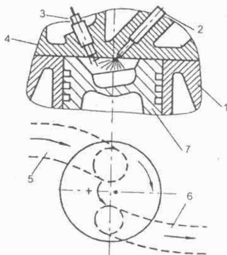
Hình 10-2. Phương pháp hình thành khí hỗn hợp phân lớp Ford Proco
