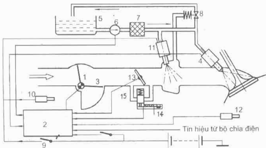
Hình 5-19. L-Electronic
