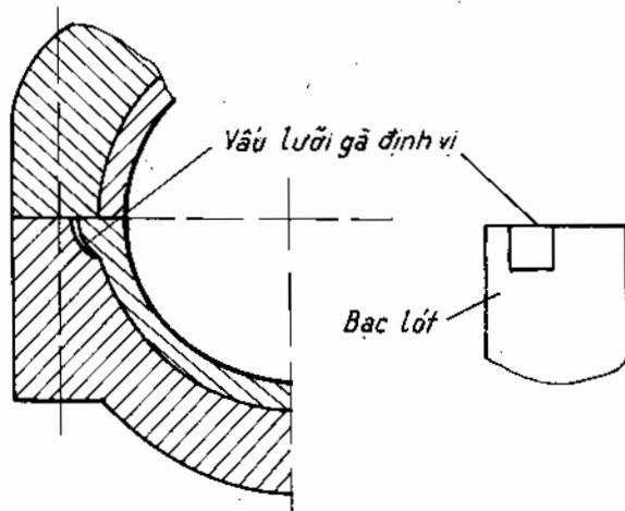
Hình 2-20. Kết cấu cố định bạc lót trên đầu to thanh truyền
