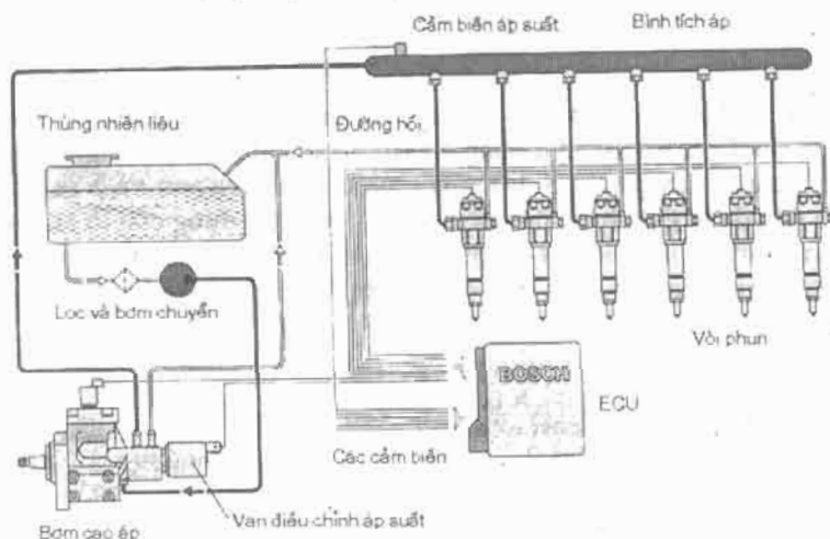
Hình 5-26. Sơ đồ hệ thống nhiên liệu tích áp
