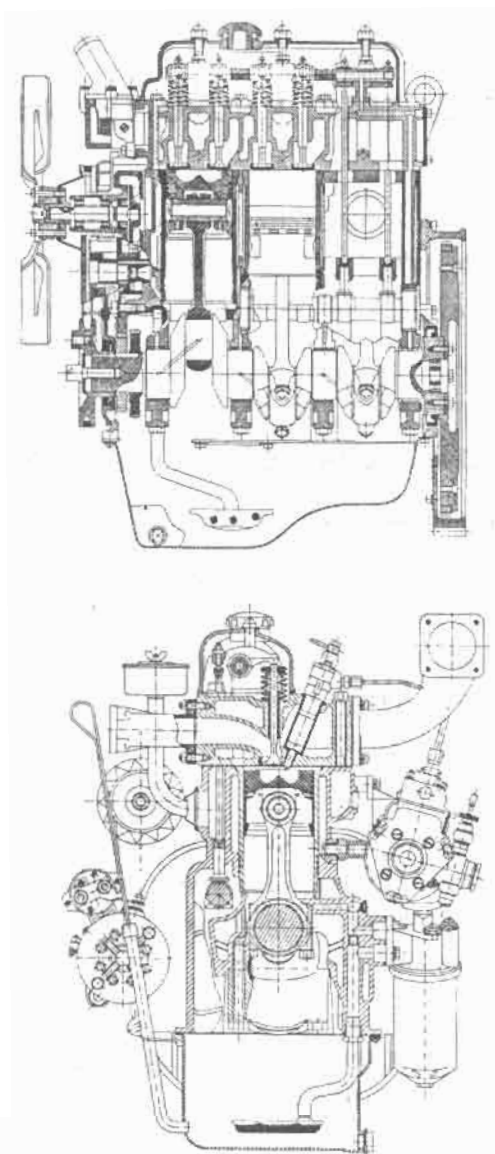
Hình 2-0. Mặt cắt dọc và mặt cắt ngang động cơ diesel 3 xy lanh 3DN88
