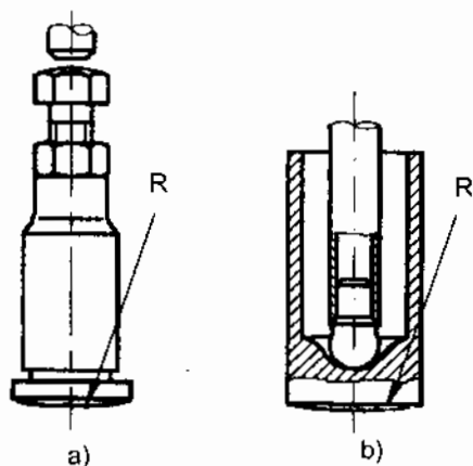
Hình 4-22. Con đội hình nấm a) và con đội hình trụ b)
