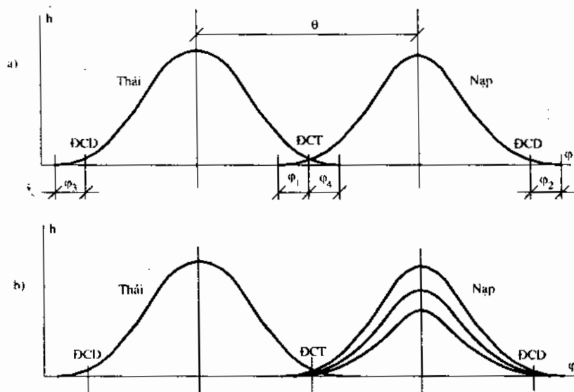
Hình 4-20. Hành trình xupap nạp và thải của một xy lanh
