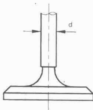
Hình 4-7. Thân xupap
