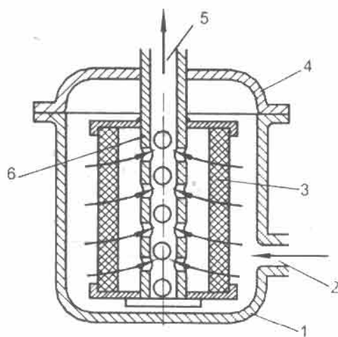
Hình 6-8. Bầu lọc thấm dùng làm lọc tinh
