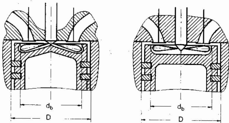
Hình 5-31. Buồng cháy thống nhất với phương pháp hỗn hợp thể tích
