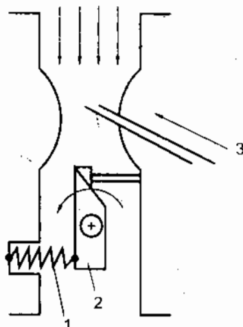
Hình 5-14. Cơ cấu hạn chế tốc độ vòng quay 1. lò xo, 2. bướm ga, 3. hệ thống chính
