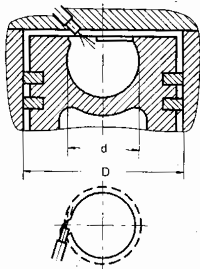
Hình 5-33. Buồng cháy hỗn hợp màng
