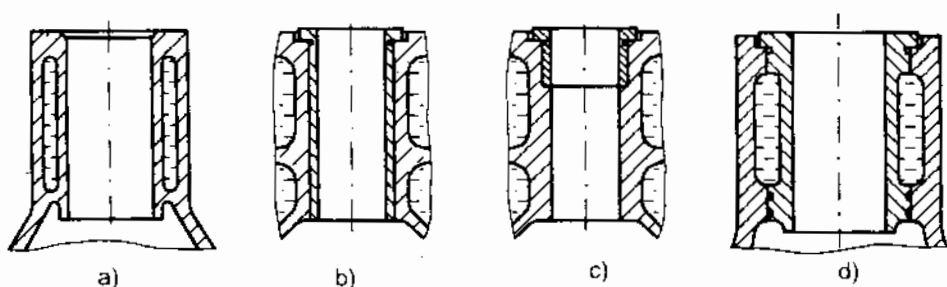
Hình 3-5. Các loại xylan a) thân xylan, b) và c) lót xylan khô, d) lót xylan ướt
