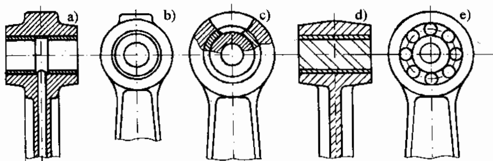
Hình 2-18. Kết cấu đầu nhỏ thanh truyền
