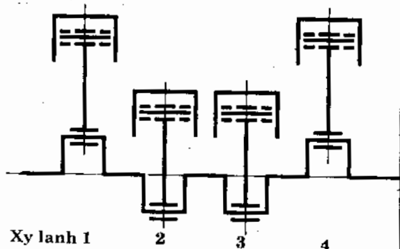
Hình 1-12. Trục khuỷu của động cơ 4 kỳ, 4 xylanh
