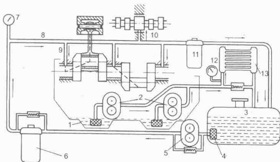
Hình 6-2. Hệ thống bôi trơn cacte khô
