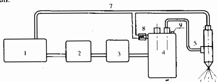
Hình 5-21. Sơ đồ hệ thống nhiên liệu động cơ diesel
