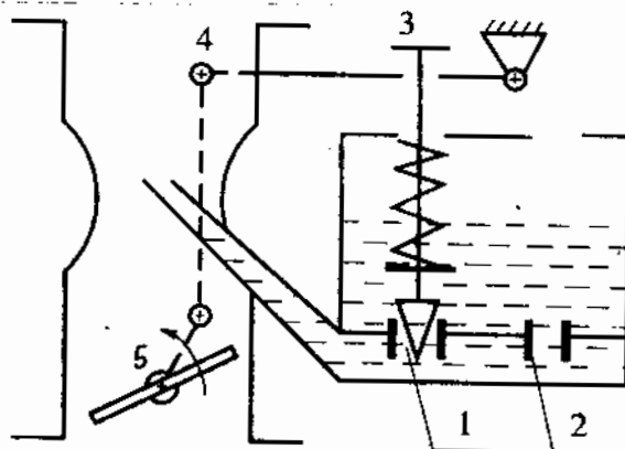
Hình 5-9. Hệ thống làm đậm cơ khí
