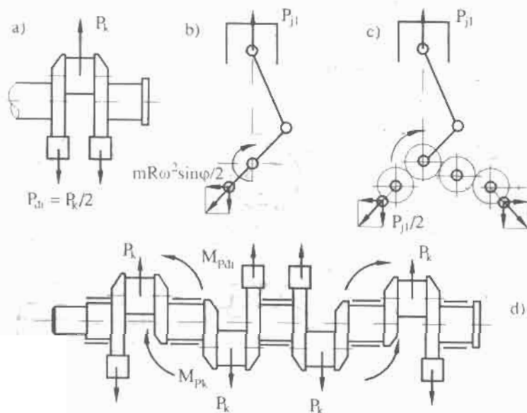
Hình 2-30. Vai trò của đối trọng
