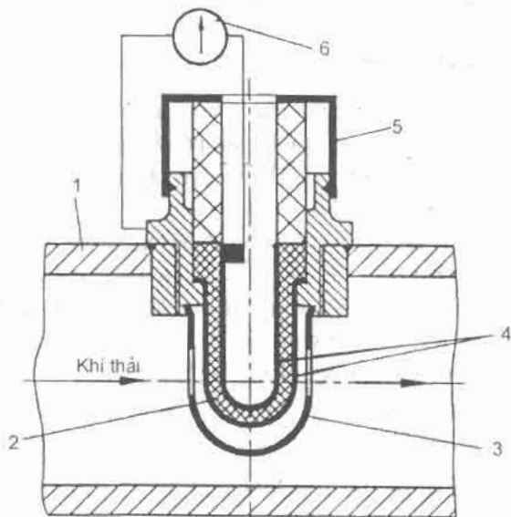
Hình 10-5. Cảm biến thành phần hệ số dư lượng không khí \lambda
