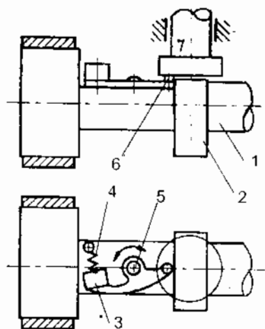
Hình 9-5. Cơ cấu giảm áp tự động 1. trục cam phối khí, 2. cam, 3. quả văng, 4. lò xo, 5. chốt quay, 6. vấu nâng, 7. con đội
