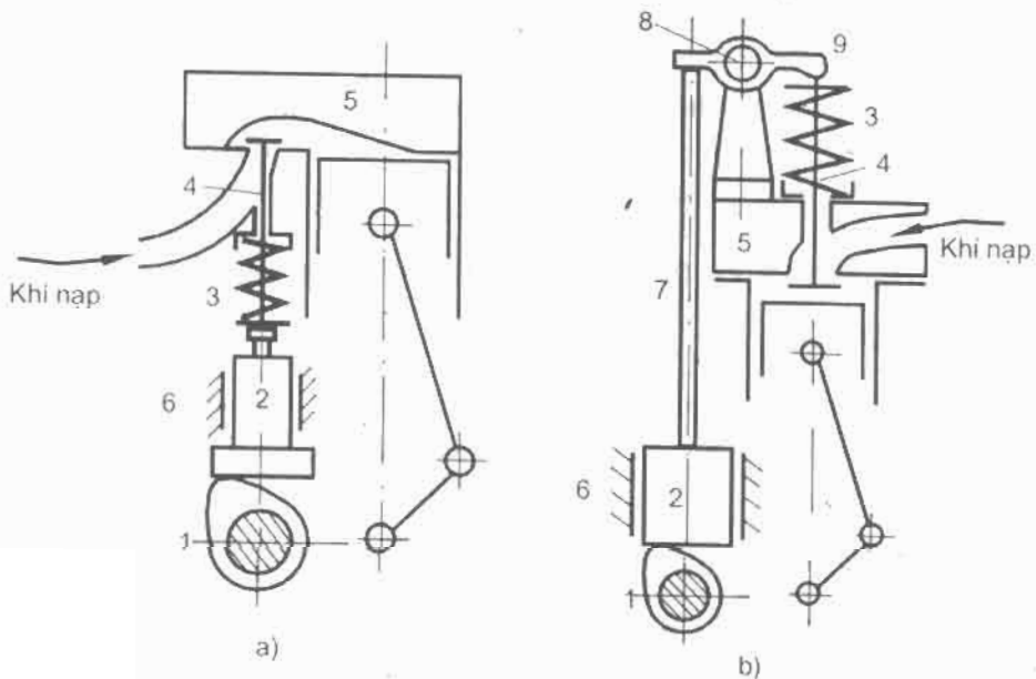
Hình 4-1. Cơ cấu phối khí dùng xupap
