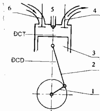
Hình 1-4. Sơ đồ động cơ
