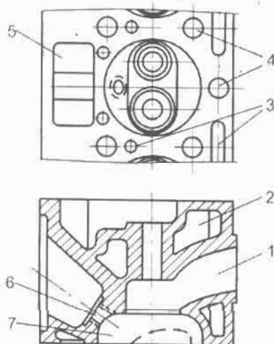
Hình 3-7. Buồng cháy bán cầu trong động cơ xăng 1. đường thải (hoặc nạp), 2. khoang nước làm mát, 3. lỗ thông nước lên nắp máy, 4. lỗ gugiông, 5. khoang lắp đưa dây, 6. khoang lắp bugi, 7. buồng cháy
