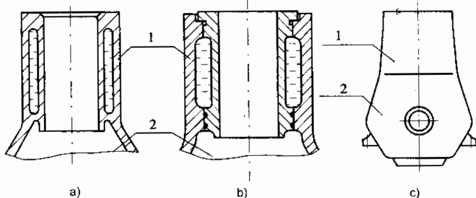
Hình 3-2. Thân máy kiểu thân xylanh - hộp trục khuỷu 1. thân xylanh, 2. hộp trục khuỷu
