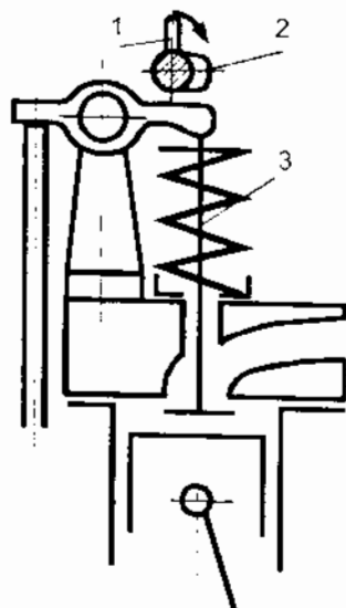
Hình 9-4. Cơ cấu giảm áp trên nắp xylanh 1. Cam, 2. tay gạt, 3. xupap tháo
