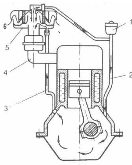
Hình 6-11. Thông gió kín (hộp trực khuỷu) 1. ống đổ dầu, 2. ống gió vào, 3. ống gió ra, 4. đường nạp, 5. bầu lọc gió, 6. đầu giữ bụi
