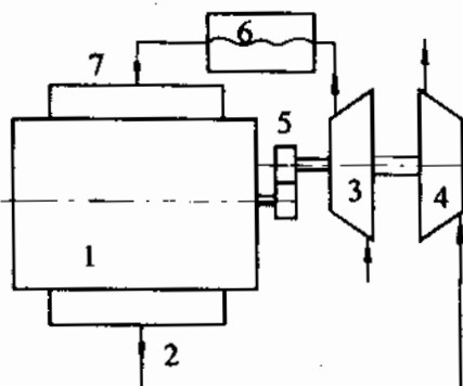
Hình 1-11. Tăng áp hỗn hợp 1. động cơ, 2. đường thải, 3. máy nén, 4. tuabin, 5. hệ truyền cơ khí, 6. bình làm mát trung gian, 7. đường nạp
