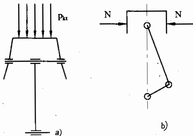
Hình 2-8. Các nguyên nhân gây bó kẹt piston
