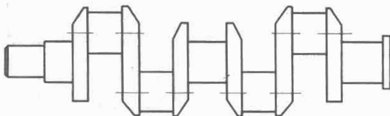
Hình 2-25. Trục khuỷu động cơ 4 kỳ, 4 xylanh, trốn cổ
