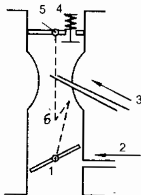
Hình 5-12. Hệ thống khởi động
