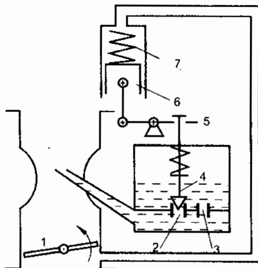
Hình 5-11. Hệ thống làm đậm chân không
