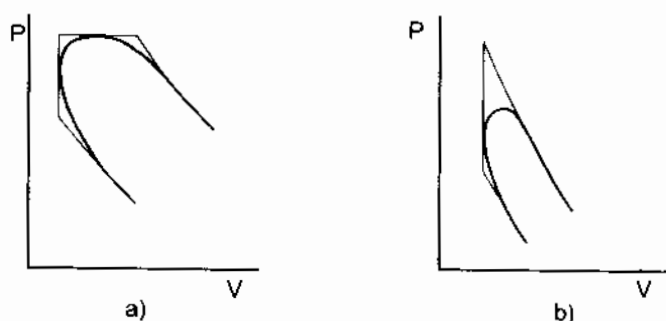
Hình 1-6. Quá trình cháy của động cơ diesel a) và động cơ xăng b)
