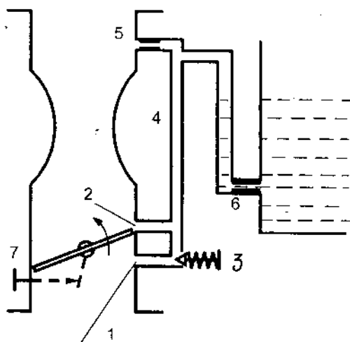
Hình 5-8. Hệ thống không tải 1. lỗ cung cấp hỗn hợp, 2. lỗ chuyển tiếp, 3. vít điều chỉnh hỗn hợp, 4. ống hỗn hợp, 5. gicơ không khí, 6. gicơ nhiên liệu, 7. vít kênh ga
