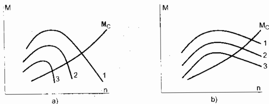
Hình 5-36. Về tính cần thiết đặt điều tốc trên động cơ diesel a) động cơ xăng, b) động cơ diesel, 1. tải lớn, 2. tải trung bình, 3. tải nhỏ
