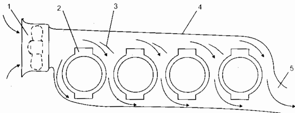
Hình 7-8. Hệ thống làm mát bằng không khí
