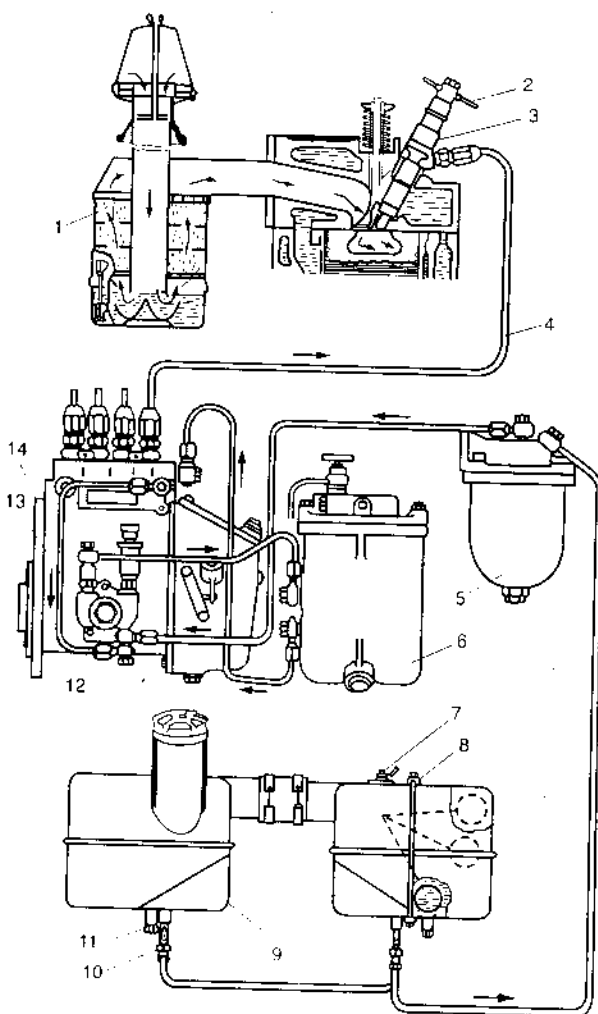
Hình 10.1. Hệ thống cung cấp nhiên liệu động cơ điêden
