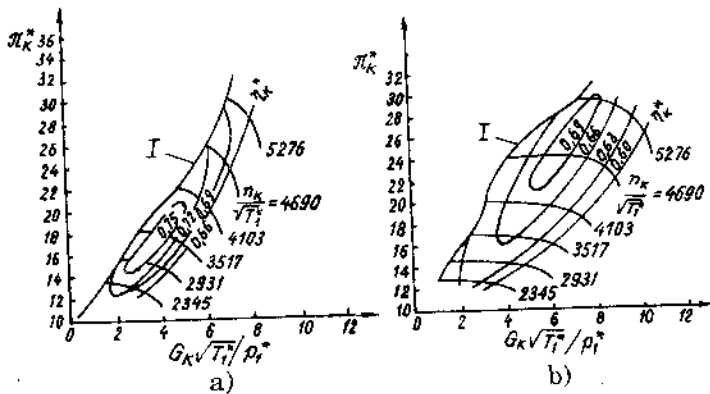
Hình 8.20. Đặc tính máy nén khí có cánh (a) và không có cánh (b), trong vành tăng áp. I - đường giới hạn ổn định.
