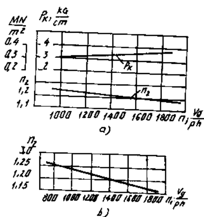
Hình 5.89. Sự thay đổi chỉ số giãn nở đa biến trung bình n_2 và áp suất cuối quá trình dẫn nở theo số vòng quay của trục khuỷu a) Động cơ Tatra - 912 ; b) Động cơ ЯМЗ-236.
