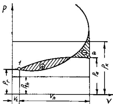
Hình 5.94. Diễn biến quá trình thải trong động cơ bốn kỳ tăng áp, khi p_r < p_k .
