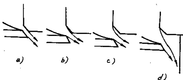
Hình 5.19. Dòng chảy qua khe hở hình vành khuyên quanh tán xupáp.
