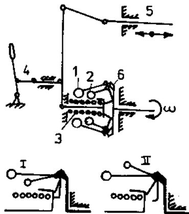
Hình 12.11. Bộ điều tốc hai chế độ có hai cặp quả văng cùng tác dụng lên một lò xo 1 - quả văng lớn ; 2 - quả văng nhỏ ; 3 - lò xo ; 4 - tay gạt ; 5 - bơm cao áp ; 6 - chốt hãm. I - quả văng lớn tỳ lên chốt hãm ; II - chuyển động của quả văng nhỏ.
