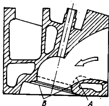
Hình 5.20. Phương án thay đổi cấu tạo đường thông vào cửa nạp của hãng Fort Mark
