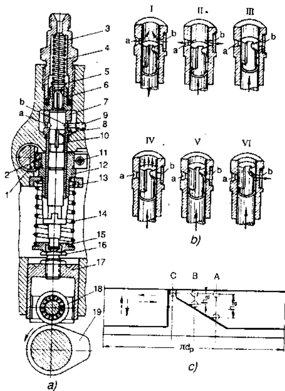
Hình 10.3. Bơm Bosch
