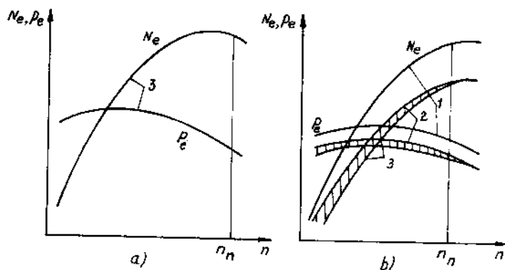
Hình 11.14. Đặc tính tốc độ a) Động cơ xăng dùng chế hòa khí; b) Động cơ diesel 1 - đặc tính ngoài tuyệt đối; 2 - đặc tính nhà khối đen; 3 - đặc tính ngoài.
