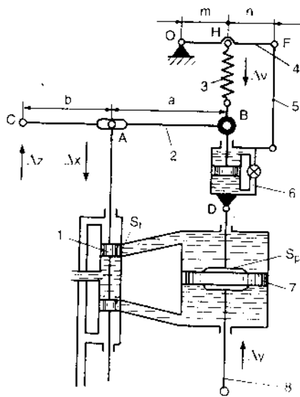
Hình 12.19. Bộ khuếch đại thủy lực có liên hệ ngược hỗn hợp
