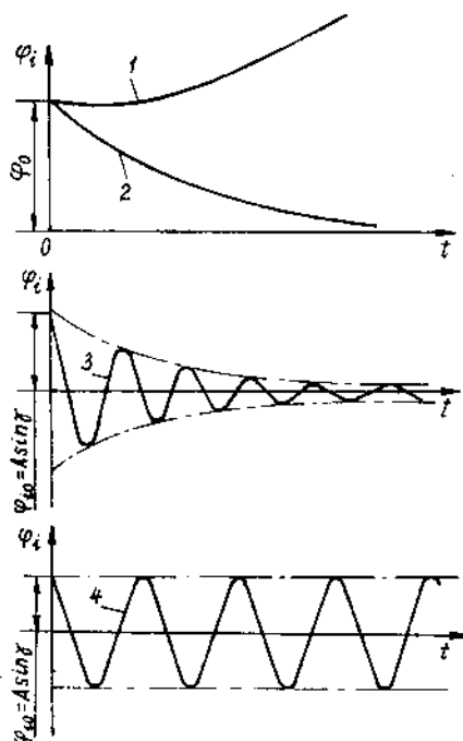
Hình 12.41. Các thành phần của quá trình chuyển tiếp 1 - hội tụ không dao động ; 2 - phân kỳ không dao động ; 3 - hội tụ dao động ; 4 - phân kỳ dao động.
