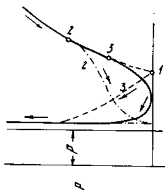
Hình 5.15. Vị trí mở xupáp xả.
