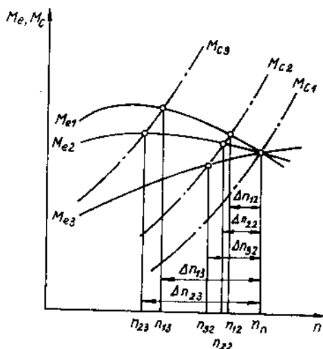
Hình 11.33. Ảnh hưởng của sự biến thiên của mômen theo tốc độ n tới tính ổn định của chế độ làm việc.
