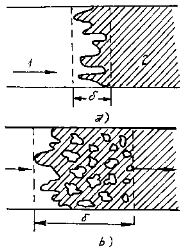
Hình 5.53. Mặt tiên phong của màng lửa chảy rối a) Mặt nhấp nhô; b) Các khối hòa khí phân tán; 1 - hòa khí mới; 2 - sản vật cháy.
