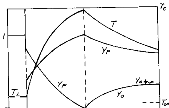
Hình 5.56. Phân bố nhiệt độ và nồng độ trong ngọn lửa khuếch tán.
