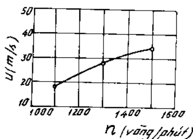
Hình 5.72. Ảnh hưởng của tốc độ động cơ n tới tốc độ lan truyền màng lửa u .
