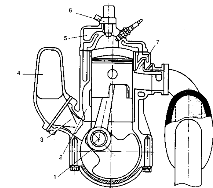
Hình 7.8. Động cơ Suzuki hai kỳ dùng vòi phun điều khiển khí nén ORBITAL.
