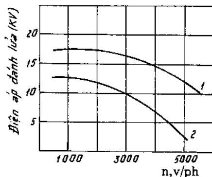
Hình 5.71. Đặc tính điện áp đánh lửa 1 - đánh lửa bán dẫn ; 2 - đánh lửa truyền thống.
