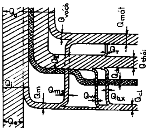
Hình 6.15. Sơ đồ cân bằng nhiệt của động cơ
