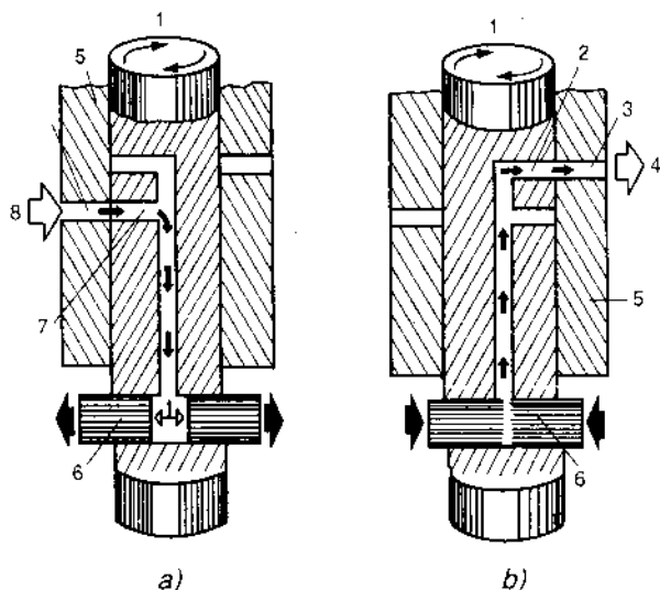
Hình 10.11. Nạp và bơm nhiên liệu trong bơm phân phối 1 - rôto ; 2 - lỗ phân phối ; 3 - lỗ ra ; 4 - đầu tới vòi phun ; 5 - xilanh ; 6 - pittông ; 7 - đường nạp ; 8 - cửa nạp ; 9 - lỗ định lượng.
