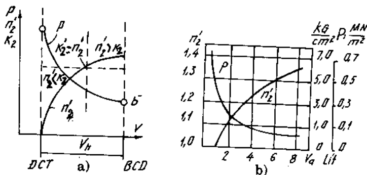
Hình 5.88. Diễn biến thực tế của áp suất p và chỉ số giãn nở n_2 trong quá trình dẫn nở
