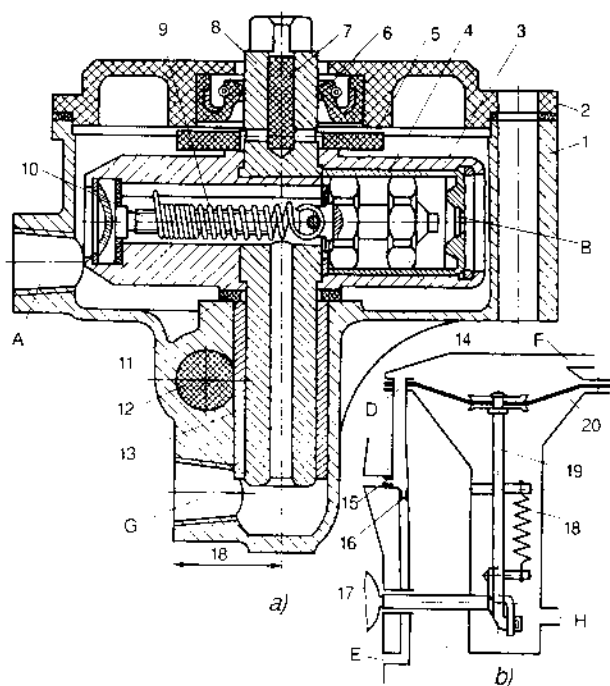
Hình 9.30. Bộ hạn chế tốc độ kiểu ly tâm
