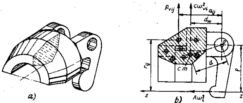
Hình 12.28. Phương pháp cắt lát quả văng để tính lực duy trì a) Cắt quả văng thành các lát mỏng ; b) Chia mỗi lát thành các hình đơn giản.
