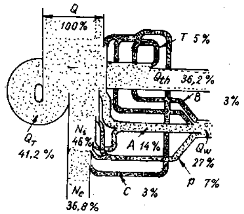
Hình 8.7. Cân bằng nhiệt động cơ tăng áp tua bin khí ở toàn tải
