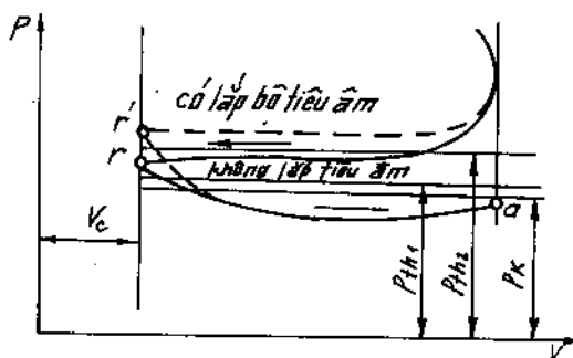
Hình 5.8. Ảnh hưởng của bình tiêu âm trên ống thải tới áp suất khí sót p_r và áp suất trên đường thải p_{br} .
