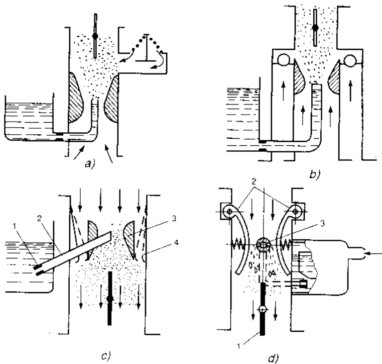
Hình 9.15. Các phương án giảm độ chân không \Delta P_h ở họng : a, b, c) Dùng van phụ đi tắt ; 1 - jiclor, 2 - vòi phun ; 3 - họng ; 4 - lò xo ; d) Thay đổi tiết diện họng ; 1 - bướm ga ; 2 - vòi phun ; 3 - họng.
