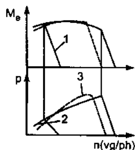
Hình 10.22. Mối quan hệ giữa p , M_e với n
