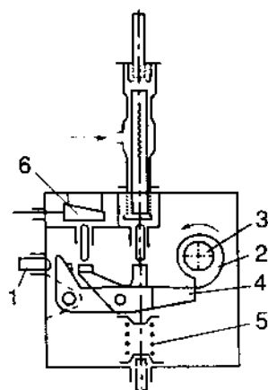
Hình 10.2. Sơ đồ bơm cao áp thay đổi hành trình toàn bộ của pittông, dẫn động bằng lò xo.
