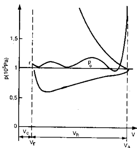
Hình 5.26. Đồ thị công vùng thấp áp của quá trình thay đổi môi chất.
