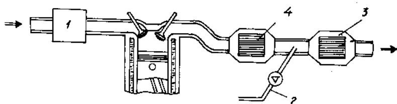
c) Bộ xúc tác 3 chức năng
